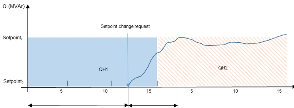
Figuur 3: Voorbeeld van de berekening van \Delta Q_{req} voor 2 kwartieren waarin een aanvraag tot wijziging van de Referentiewaarde is doorgegeven nadat binnen het eerste kwartier 10 minuten verstreken zijn
