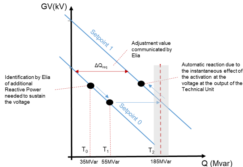
Figuur 4: Voorbeeld van een aanvraag van Elia tot wijziging van de Referentiewaarde
