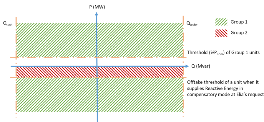
Figuur 5: Technische Eenheden van Groep 1 en Groep 2
