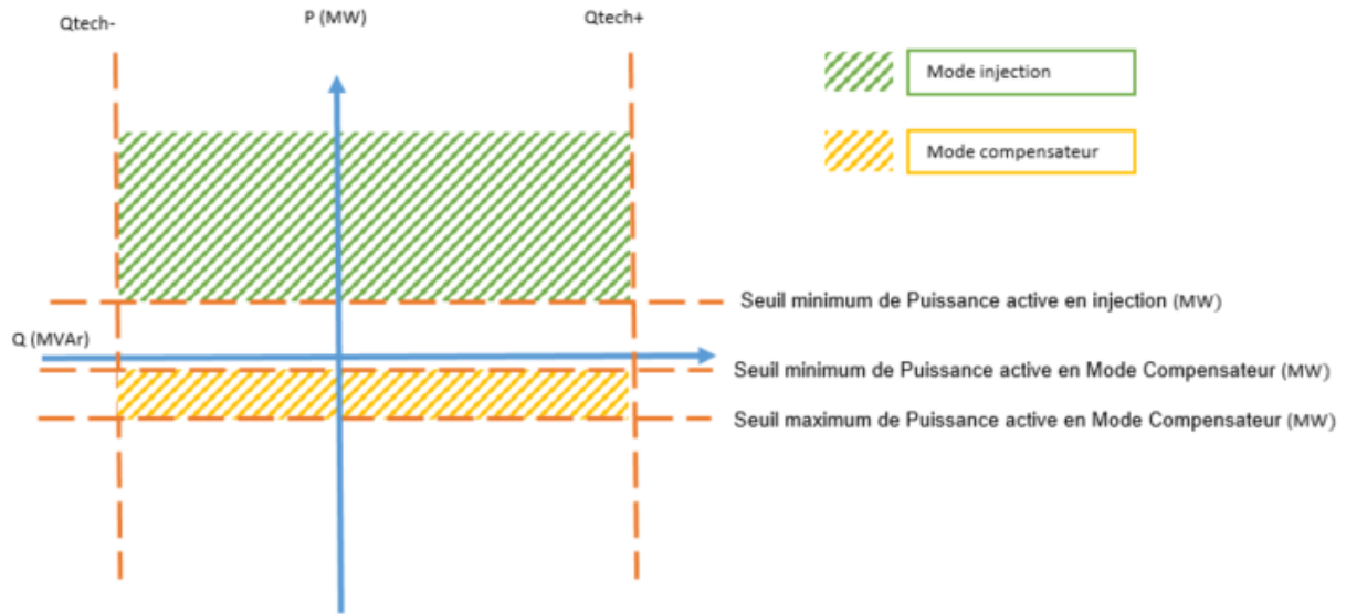
Illustration 7 : Unité Technique capable de fournir le Service en Mode injection en injectant de l'Energie Active (option a(i)) seulement et capable de fournir le Service en Mode Compensateur (option b)
