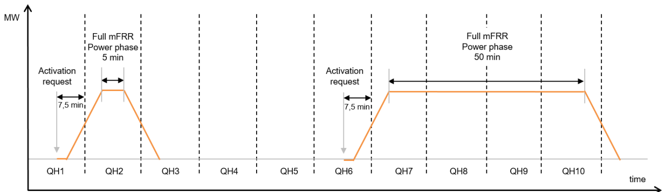
Figuur 1: Prekwalficatietestprofiel
