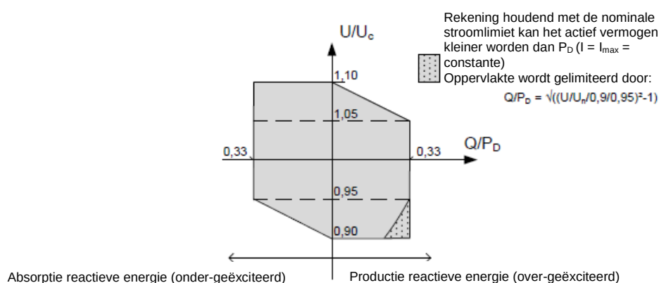
Afbeelding 12: U - Q/P_D -profiel voor PPM van het type B als weergave van de eisen inzake reactief vermogen voor andere spanningen dan 1 pu.
