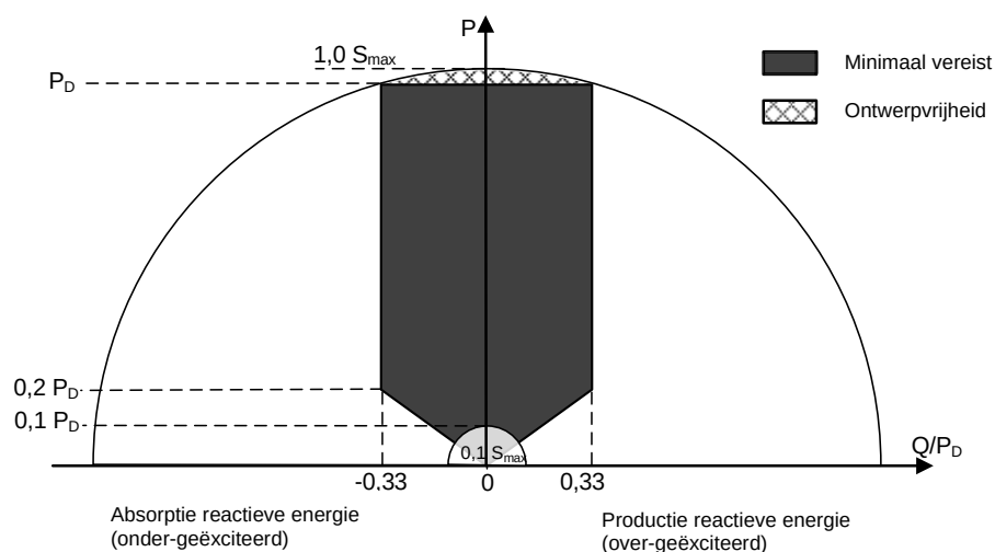
Afbeelding 7: Capaciteitscurve voor SPGM type B.
