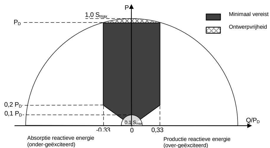
Afbeelding 11: Capaciteitscurve voor PPM type B.
