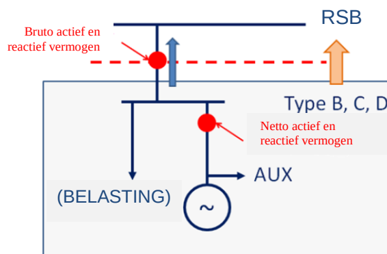
Afbeelding 6: Verduidelijking van het concept van netto en bruto meting.
