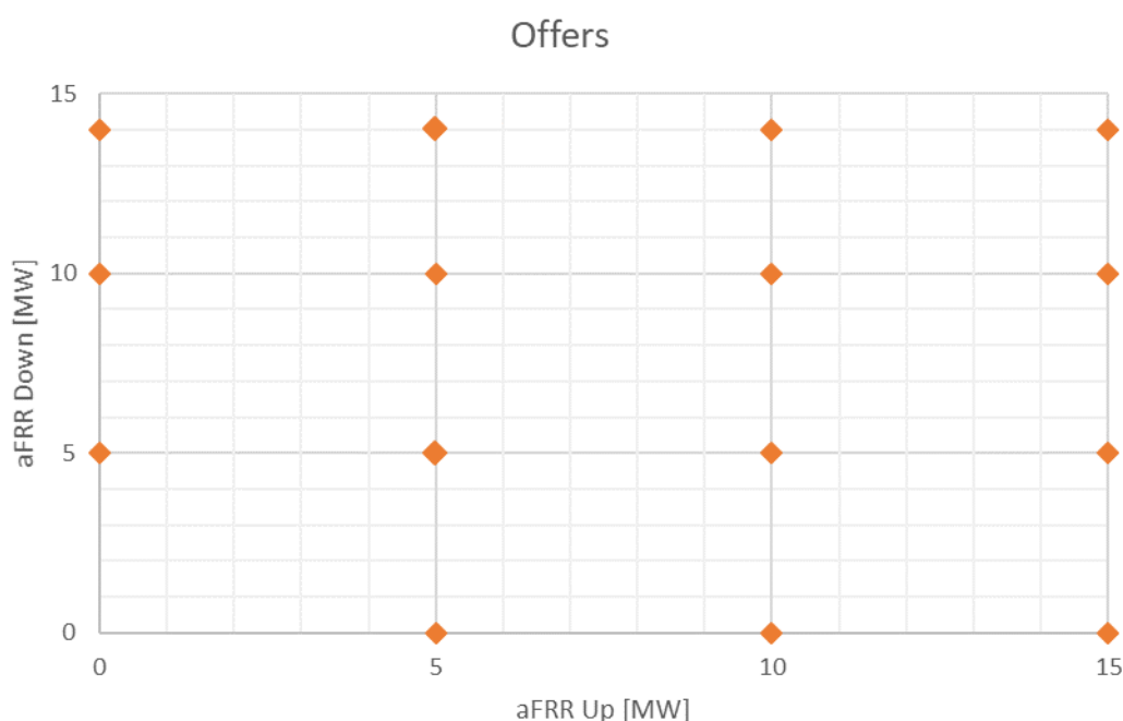
Figuur 3 - Minimumreeks aFRR-Capaciteitsbiedingen om 15 MW aFRR Up en 14 MW aFRR Down aan te bieden in een 'all-CCTU'- capaciteitsveiling
