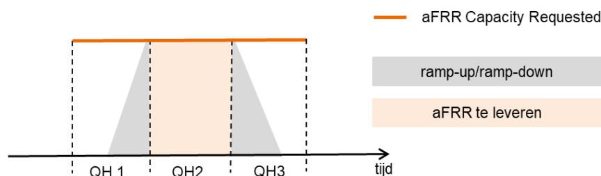
Figuur 8 - aFRR-beschikbaarheidstest
