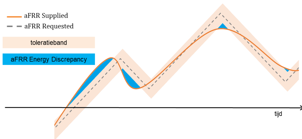
Figuur 9 - aFRR Energy Discrepancy
