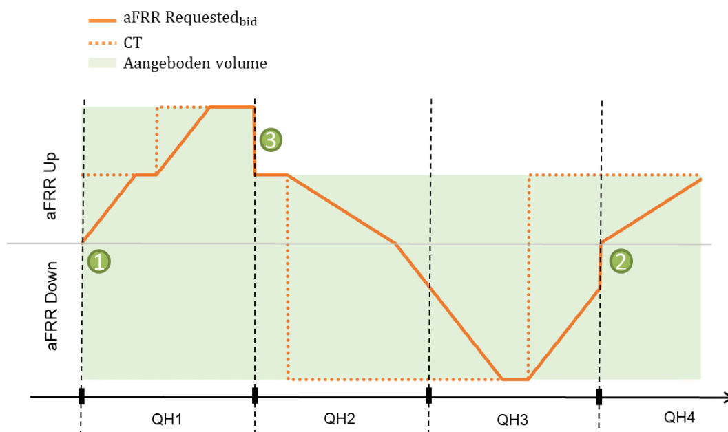
Figuur 7 - Bepaling van aFRR_{Requested_{bid}}
