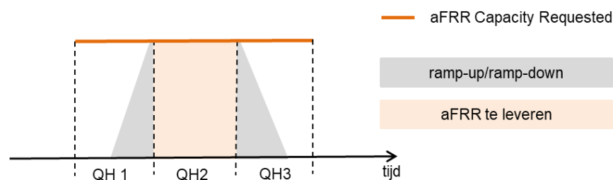
Figuur 8 - aFRR-beschikbaarheidstest
