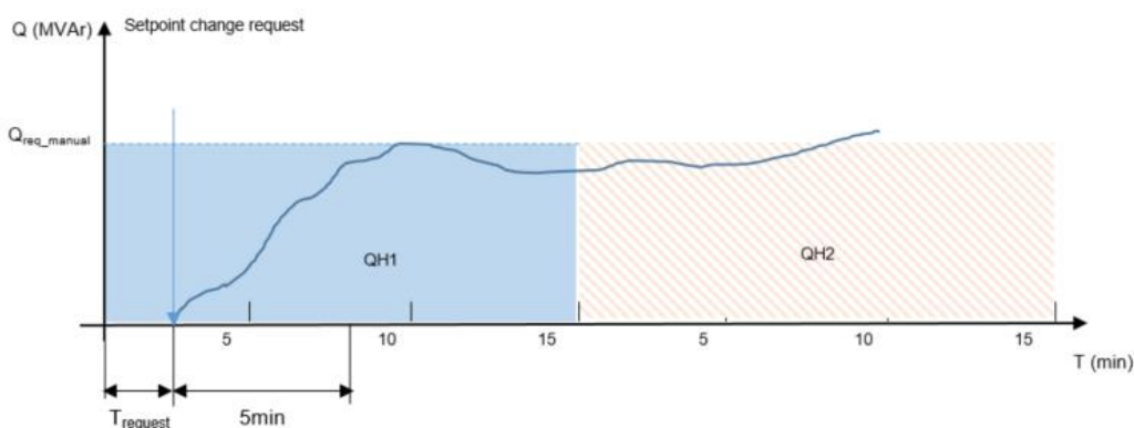
Figuur 2: Voorbeeld van de berekening van Q_{req_{rem},q} voor een kwartier waarin een aanvraag tot wijziging van de Referentiewaarde is doorgegeven voordat binnen dat kwartier 10 minuten verstreken zijn
