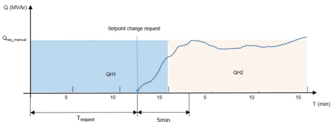
Figuur 3: Voorbeeld van de berekening van Q_{req_{rem}} voor 2 kwartieren waarin een aanvraag tot wijziging van de Referentiewaarde is doorgegeven nadat binnen het eerste kwartier 10 minuten verstreken zijn
