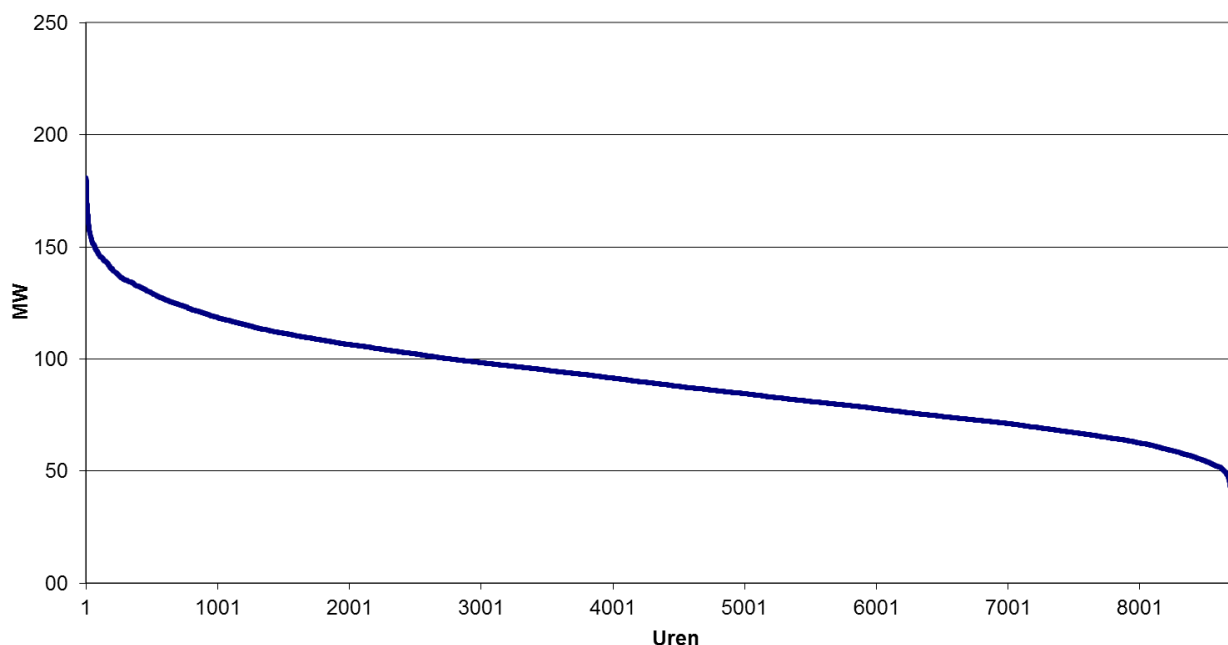
Monotone curve van de verliezen 2016 380-220-150 kV netwerk
