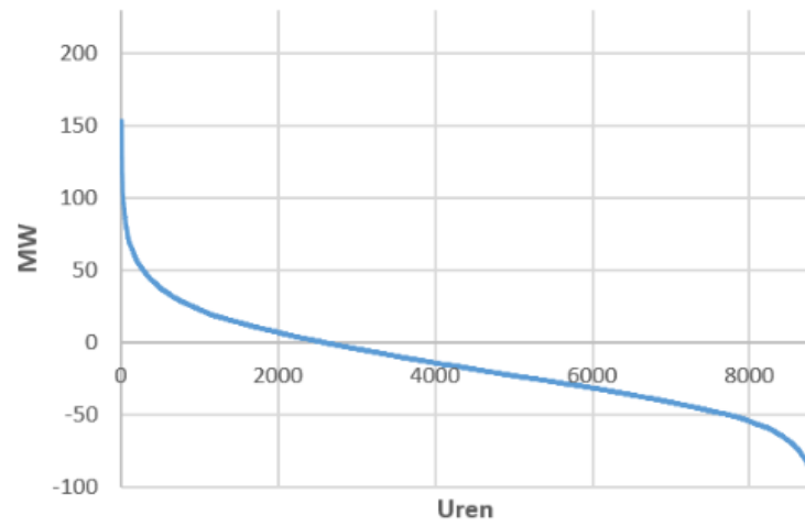
Monotone curve van het compensatietekort 2024 380-220-150 kV netwerk
