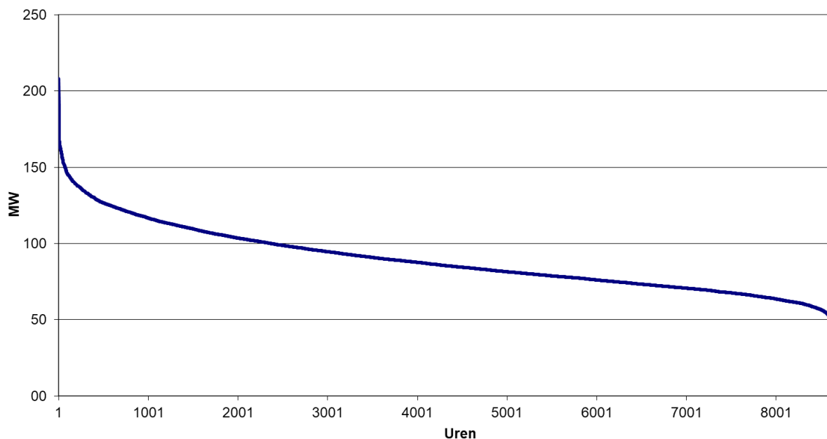
Monotone curve van de verliezen 2019 380-220-150 kV netwerk
