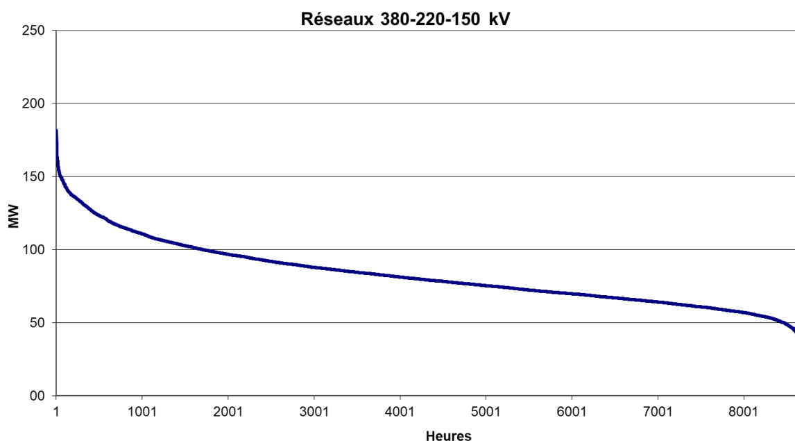
Courbe monotone des pertes 2018
