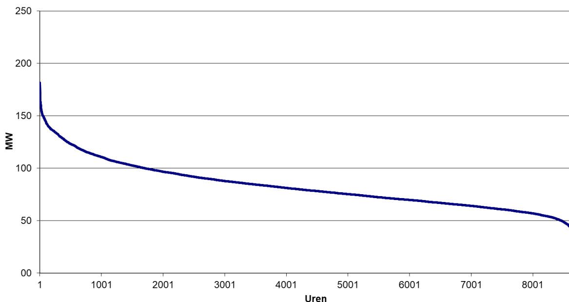
Monotone curve van de verliezen 2018 380-220-150 kV netwerk
