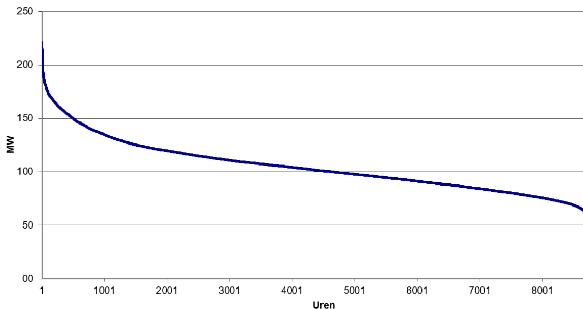
Monotone curve van de verliezen 2021 380-220-150 kV netwerk
