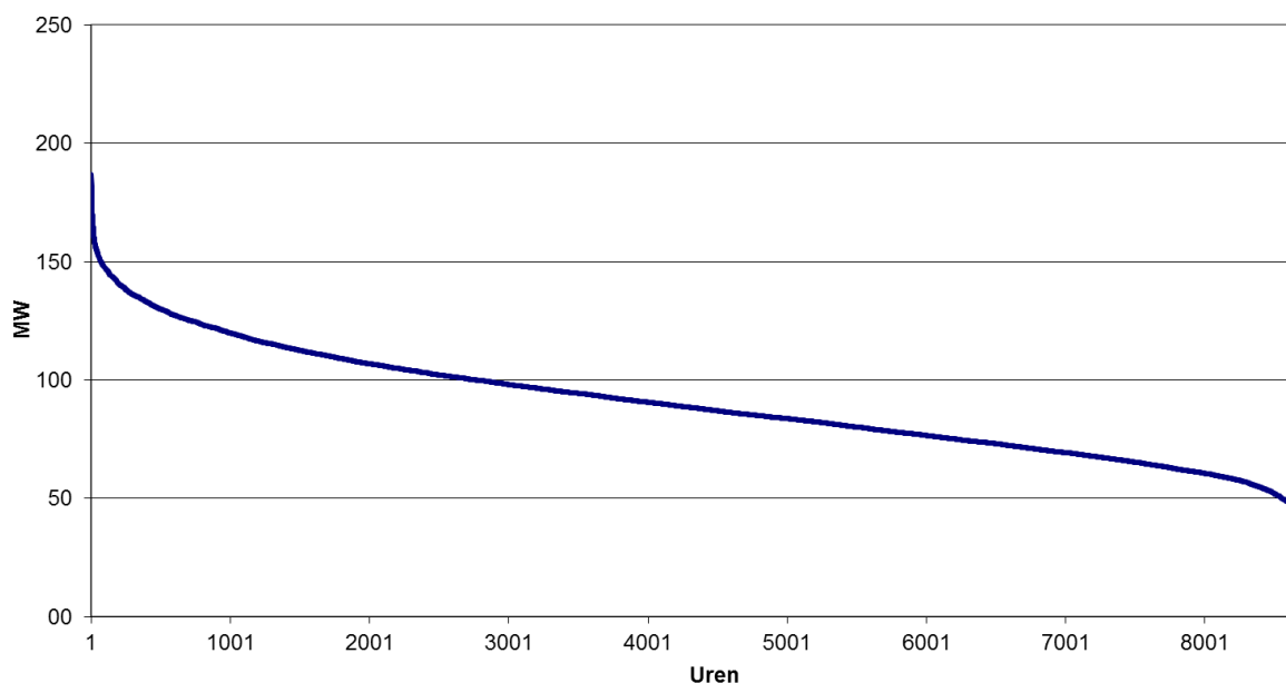
Monotone curve van de verliezen 2017 380-220-150 kV netwerk
