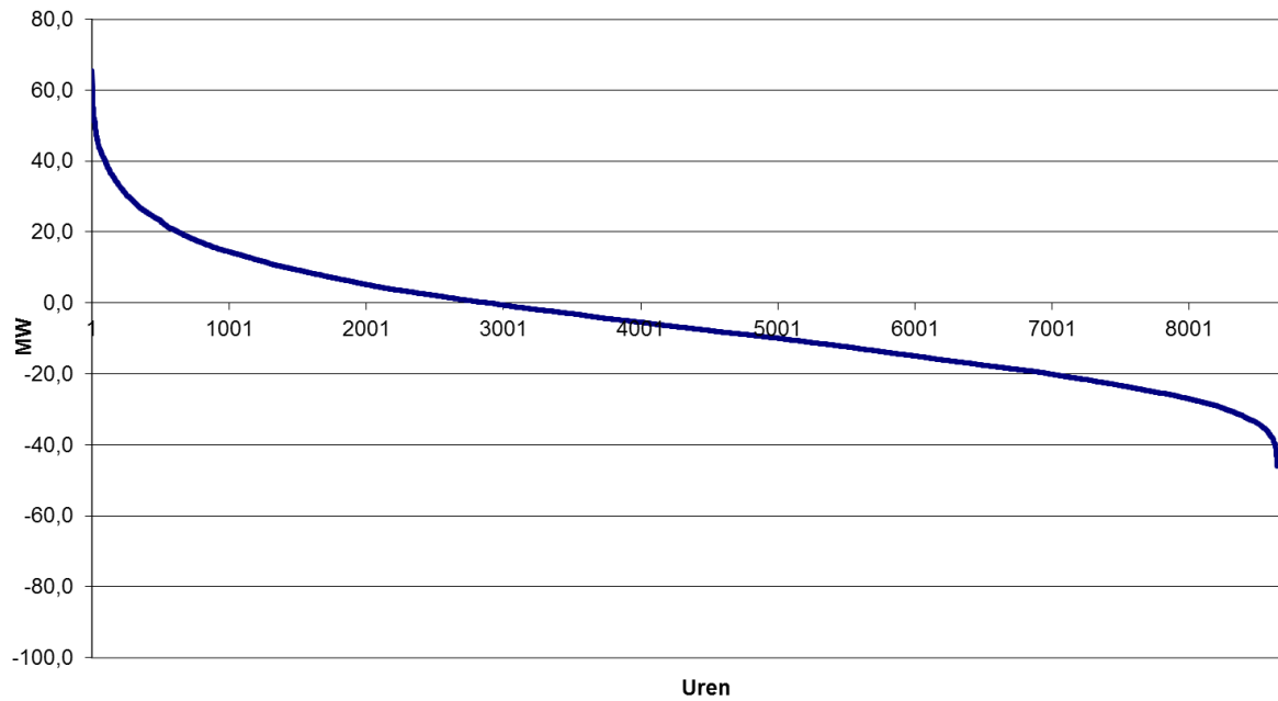
Monotone curve van het compensatietekort 2017
