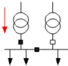
Figuur 3.3: Buiten spanning stellen van een reservetransformator
