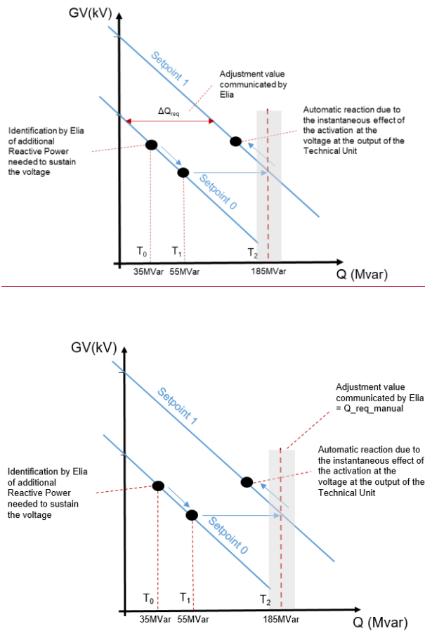
Figuur 4: Voorbeeld van een aanvraag van Elia tot wijziging van de Referentiewaarde
