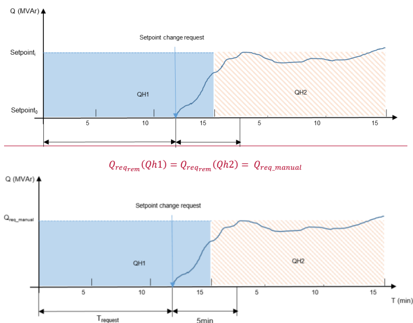
Figuur 3: Voorbeeld van de berekening van \Delta Q_{req} Q_{req_{rem}} voor 2 kwartieren waarin een aanvraag tot wijziging van de Referentiewaarde is doorgegeven nadat binnen het eerste kwartier 10 minuten verstreken zijn
