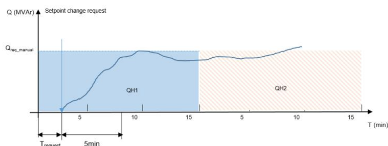
Figuur 2: Voorbeeld van de berekening van \Delta Q_{req} Q_{reqrem,q} voor een kwartier waarin een aanvraag tot wijziging van de Referentiewaarde is doorgegeven voordat binnen dat kwartier 10 minuten verstreken zijn
