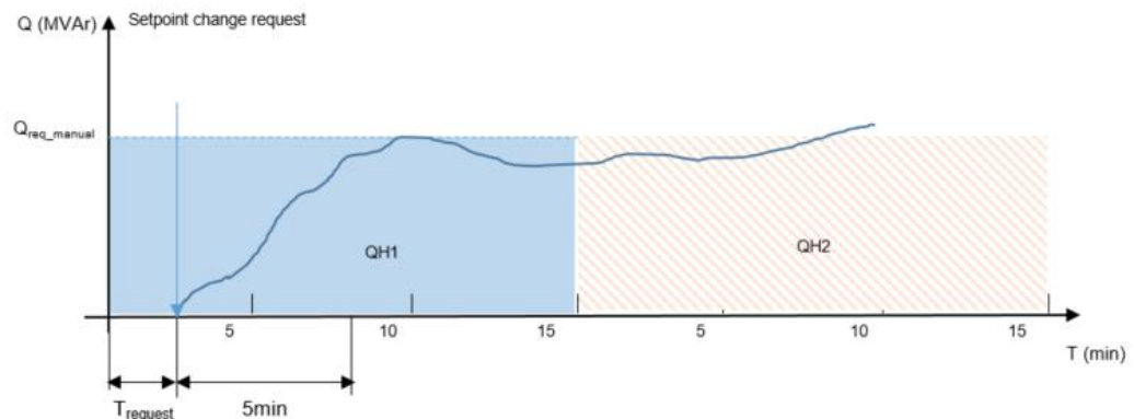
Figuur 3: Berekening van Q_{\text{req}} voor een kwartier waarin een aanvraag voor Referentiewaarde is doorgegeven voordat binnen dat kwartier 10 minuten verstreken zijn
