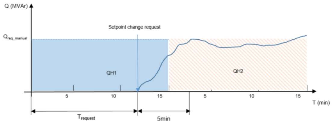
Figuur 4: Berekening van Q_{\text{req\_rem}} voor twee kwartieren waarin een aanvraag voor de Referentiewaarde is doorgegeven nadat binnen het eerste kwartier 10 minuten verstreken zijn
