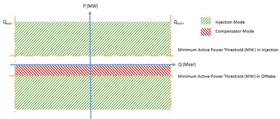
Figuur 7: Technische Eenheden in Injectiemodus en Compensatormodus
