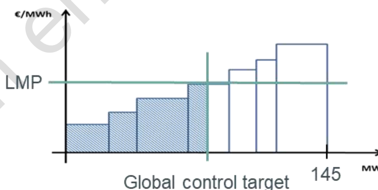
Figure 10 – Détermination du prix marginal local à partir de l'objectif de contrôle global et l'ordre de mérite (ex-post)
