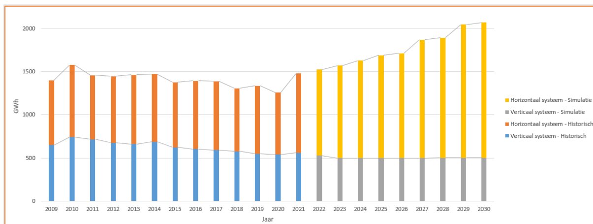
Figuur 2.14: Evolutie van de netverliezen voor het Belgische horizontale en verticale systeem.
