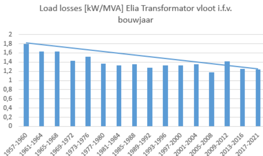
Figuur 4.5: Verliezen van de transformatoren
