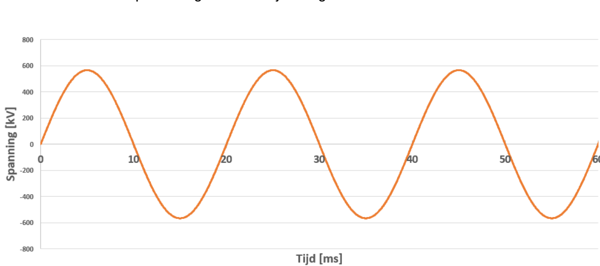
Figuur 2.9: Voorbeelden van een stabiele lijnspanning van 50 Hertz
