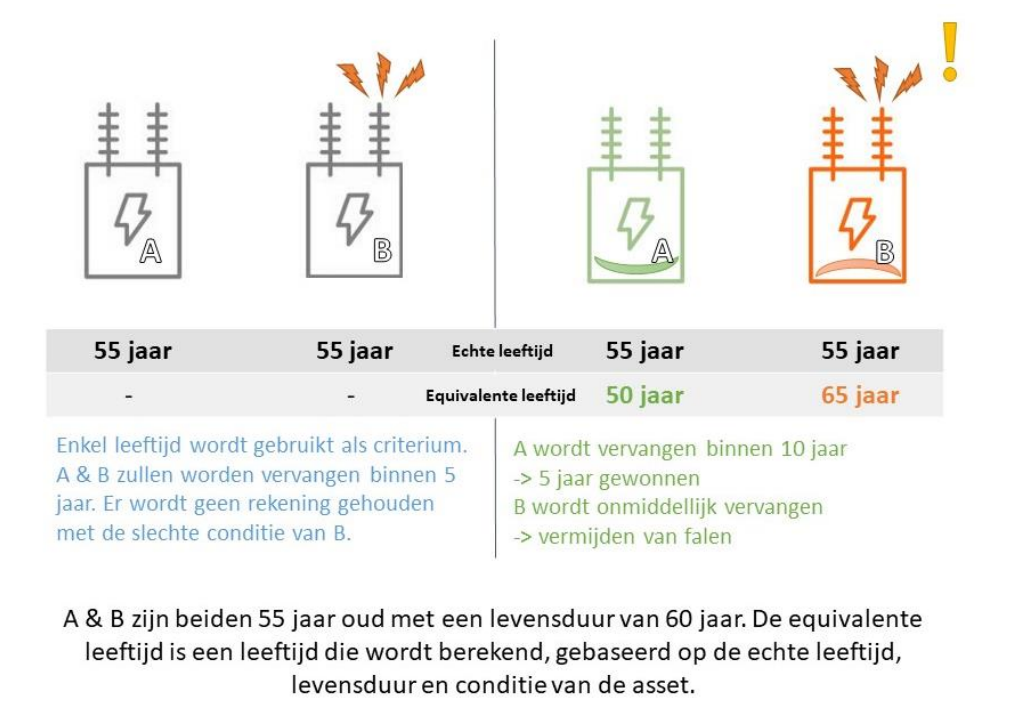
Figuur 2.10: Tijdsgebaseerd versus toestandsgebaseerd beheer van uitrustingen
