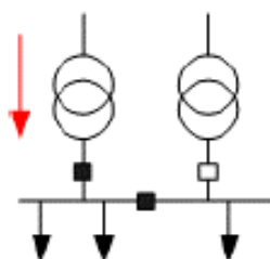
Figuur 4.3: Buiten spanning stellen van een reservetransformator
