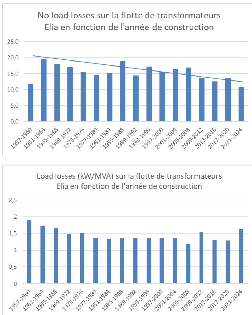
Figure 4.5: Pertes des transformateurs
