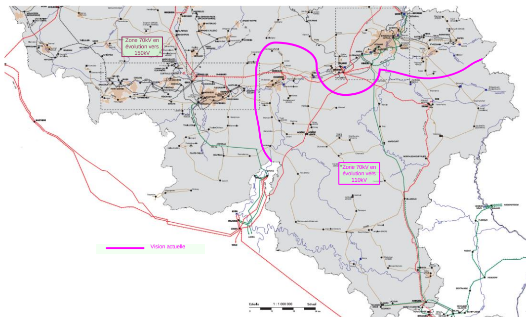
Figure 4.1 : Zones 70 kV évoluant vers 150 ou 110 kV
