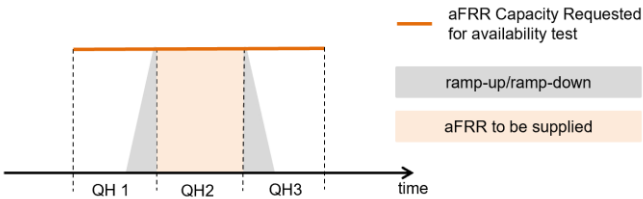
Figuur 10 - aFRR-beschikbaarheidstest
