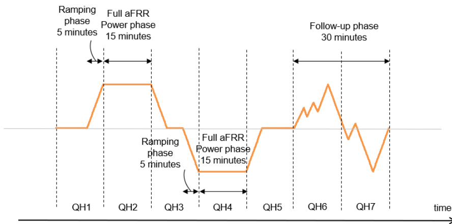
Figure 2 – Test de préqualification concernant les deux directions
