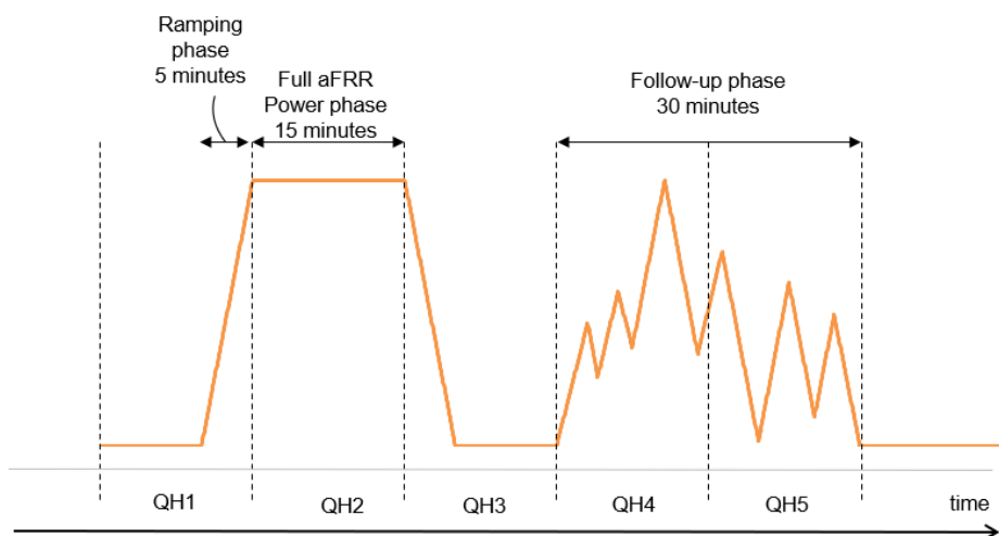
Figure 1 – Test de préqualification concernant l'aFRR Up
