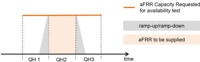
Figuur 10 - aFRR-beschikbaarheidstest
