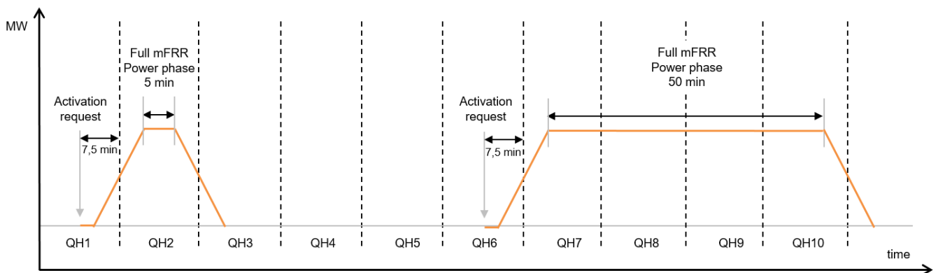
Figuur 1: Prekwalficatietestprofiel
