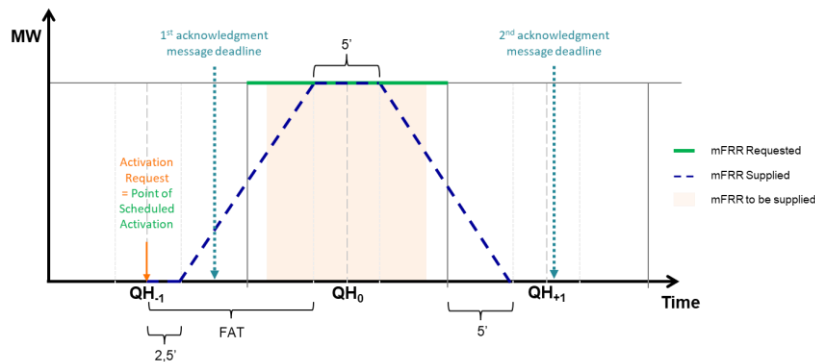
Figure 7: Activation Programmée d'une Offre d'Énergie mFRR
