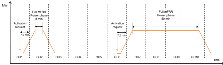
Figure 1: Profil d'un test de préqualification
