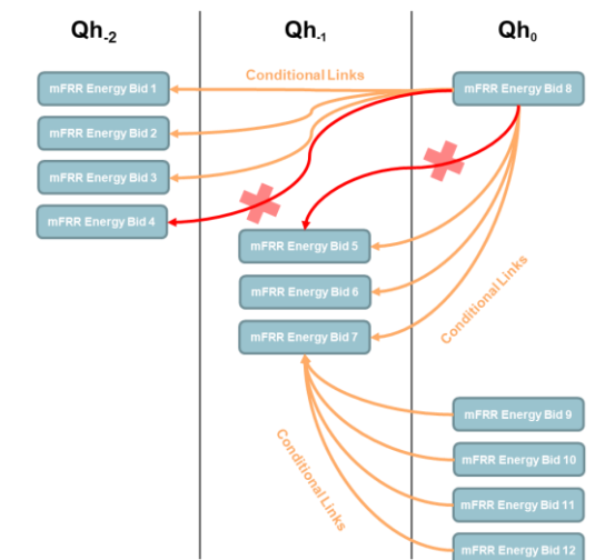
Figure 5: Illustration de liens conditionnels autorisés et non autorisés
