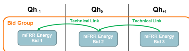
Figure 3: Illustration d'un groupe d'offres
