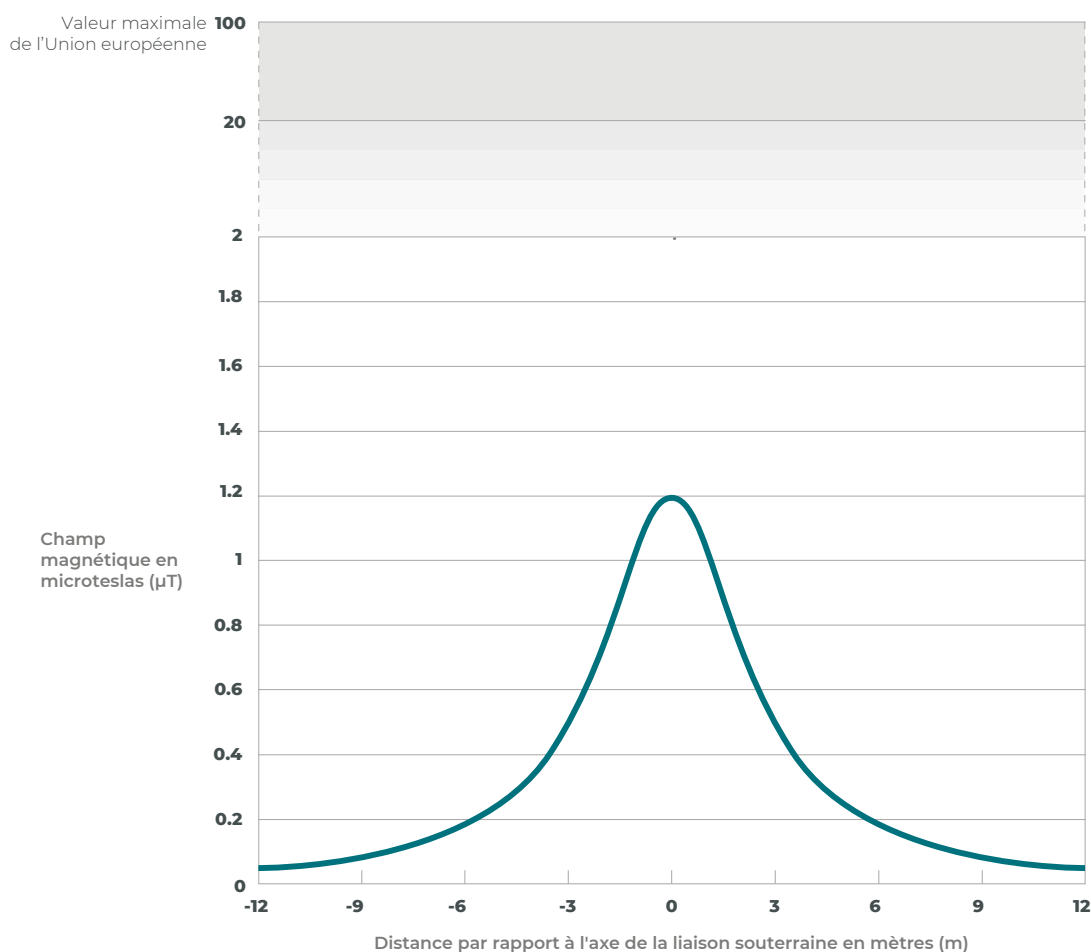
CHAMP MAGNÉTIQUE AU-DESSUS D'UNE LIAISON SOUTERRAINE (150 kV) MESURÉ À UNE HAUTEUR DE 1,5M
